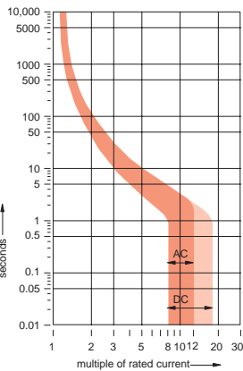
S204-K, 4 pole S203-KNA, 3P+N
