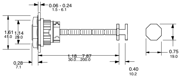
CBG reset actuator
